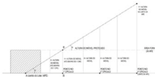
ESQUEMA ILUSTRADO DO ESCALONAMENTO NA APE (ELEVAÇÃO)
